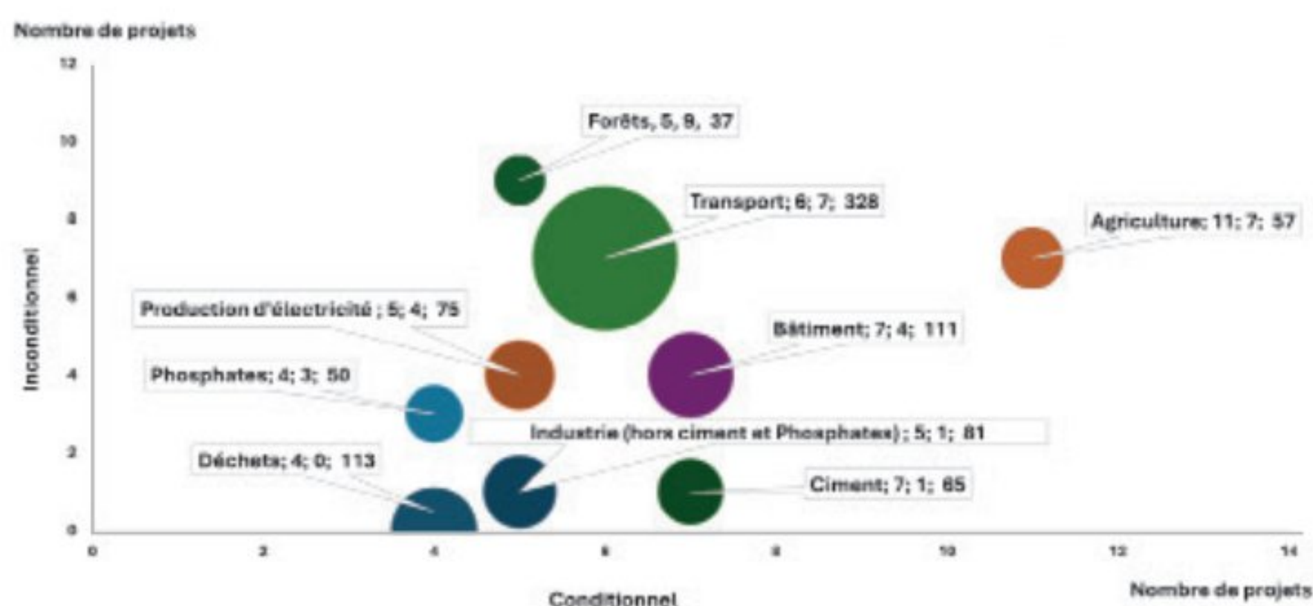
Figure 7 : Répartition des projets d'atténuation par secteur, type de conditionnalité et coût d'abattement (USD / T éq.CO 2 )
