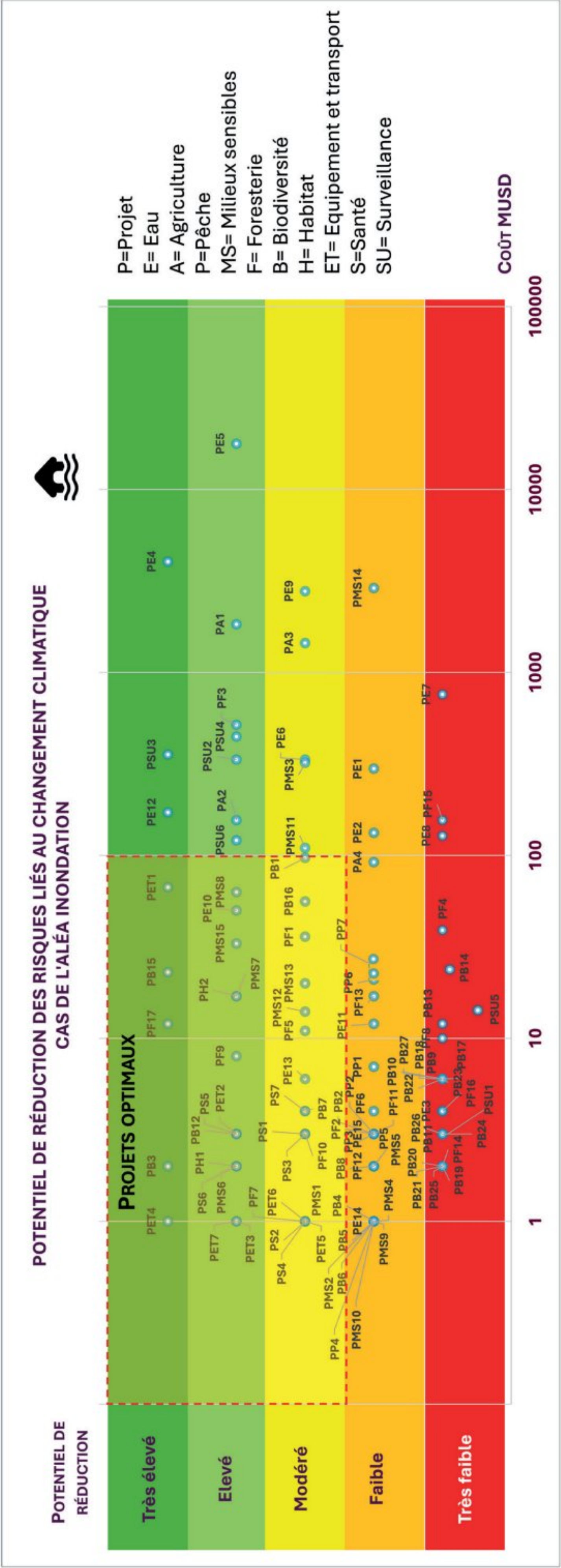
Figure 10 : Potentiel de réduction des risques liés au changement climatique, cas de l'aléa inondation
